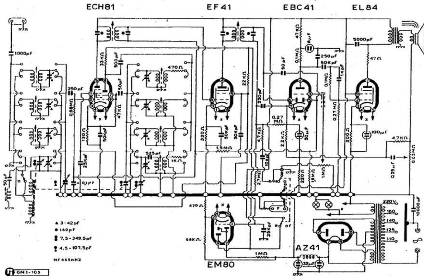
Allocchio Bacchini - Mod. 955/TA ediz. B
